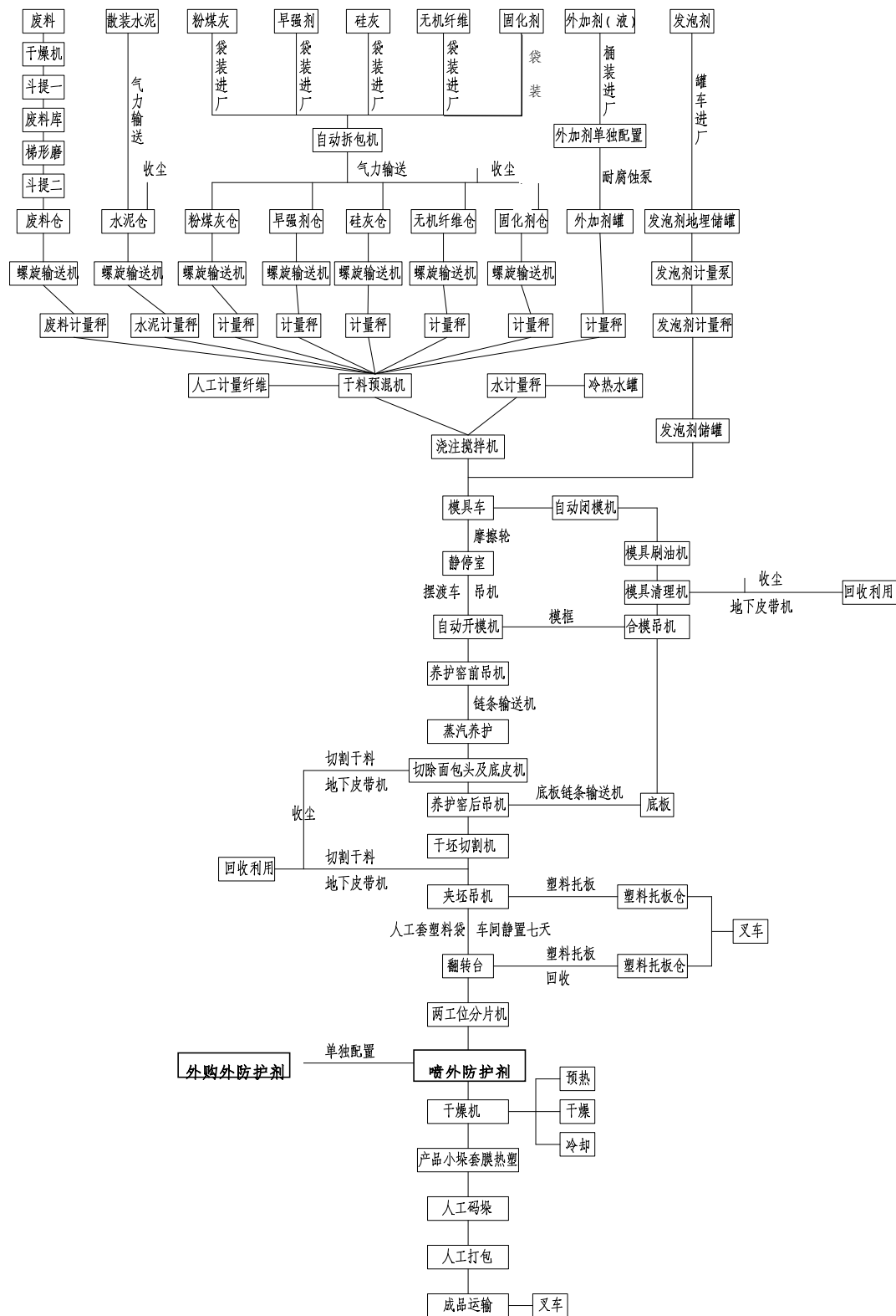
图 3-1 生产工艺流程图
