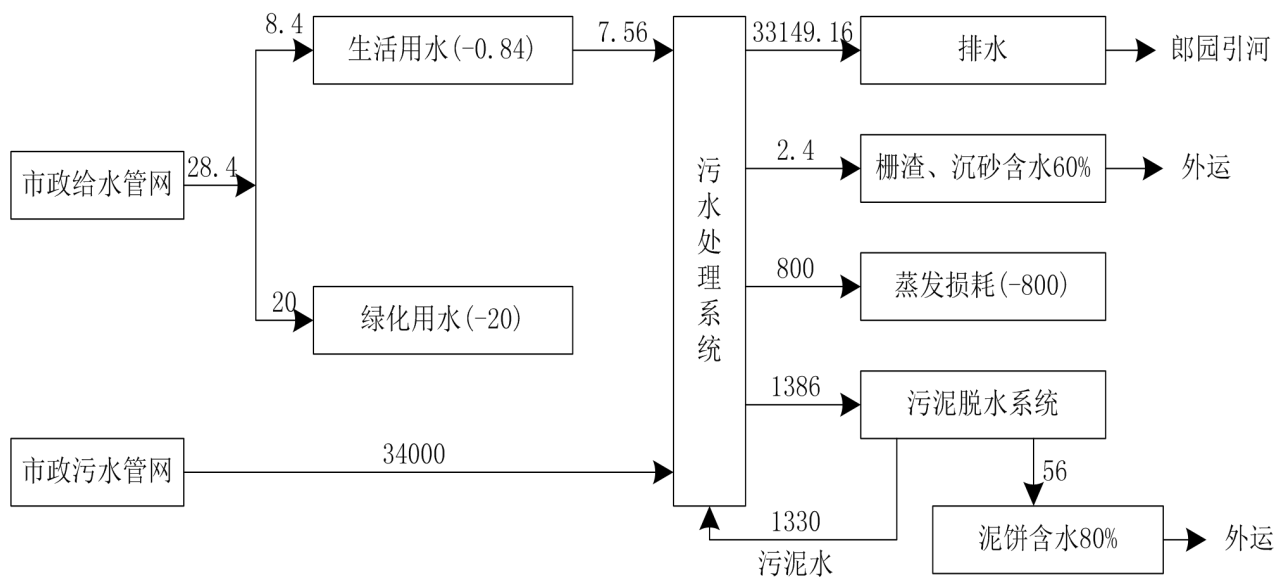
图 3-2 大双污水处理厂工程水平衡图 (单位: m³/d)
